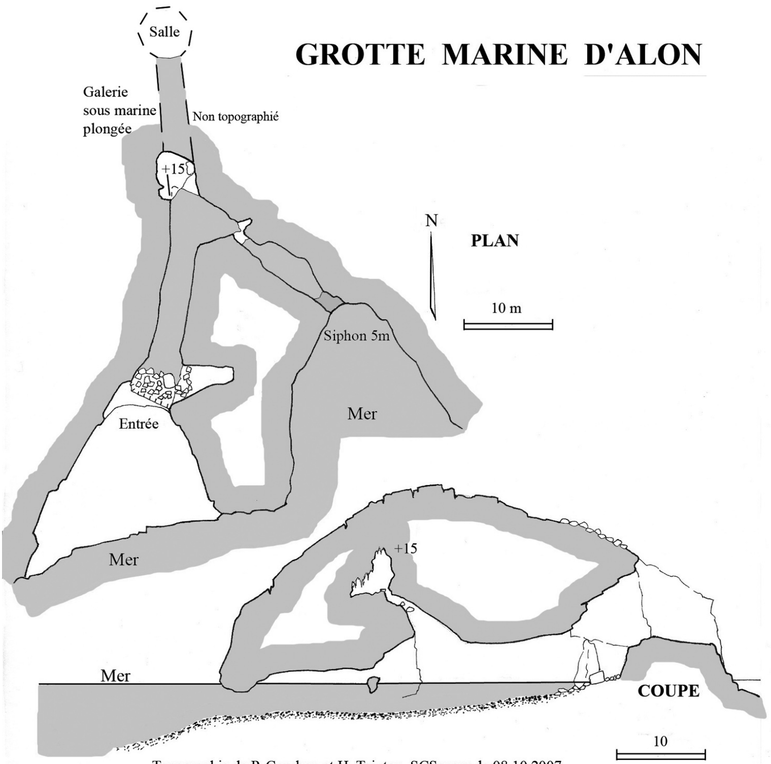
Topographie de P. Courbon et H. Tainton, SCSanary, le 08.10.2007
