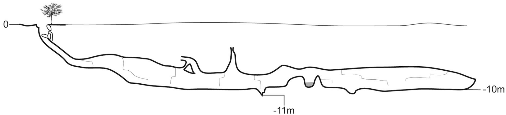
Coupe
